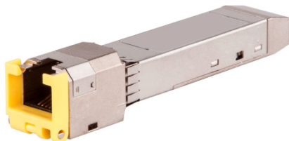
图9-4 SFP+电口光模块外观示意图
