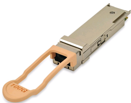
图3-1 QSFP28 光模块（MPO 接口）外观示意图
