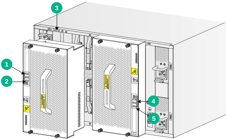
图3-5 S12504G-AF 风扇框上的网板指示灯与网板槽位对应关系
