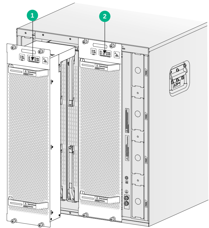
图3-4 风扇框上的网板指示灯与网板槽位对应关系（以 S12508G-AF 为例）
