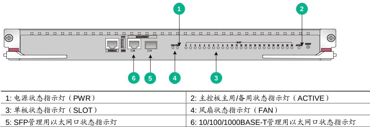
图3-2 主控板 LSXM2SUPT2 指示灯示意图
