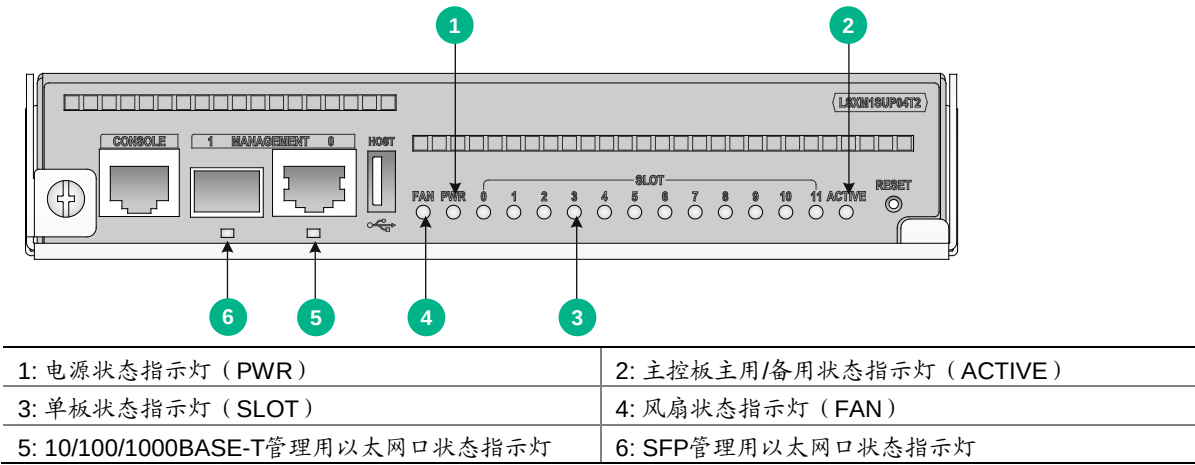
图3-3 主控板 LSXM1SUP04T2 指示灯示意图
