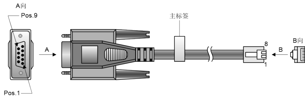
图4-1 配置电缆示意图
