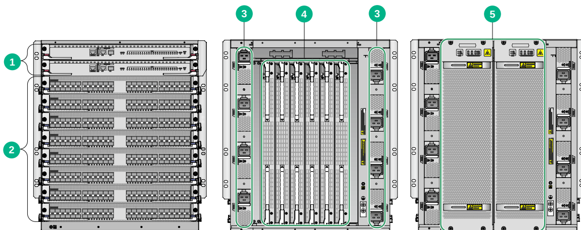
图1-2 S12508G-AF 交换机前、后面板示意图
