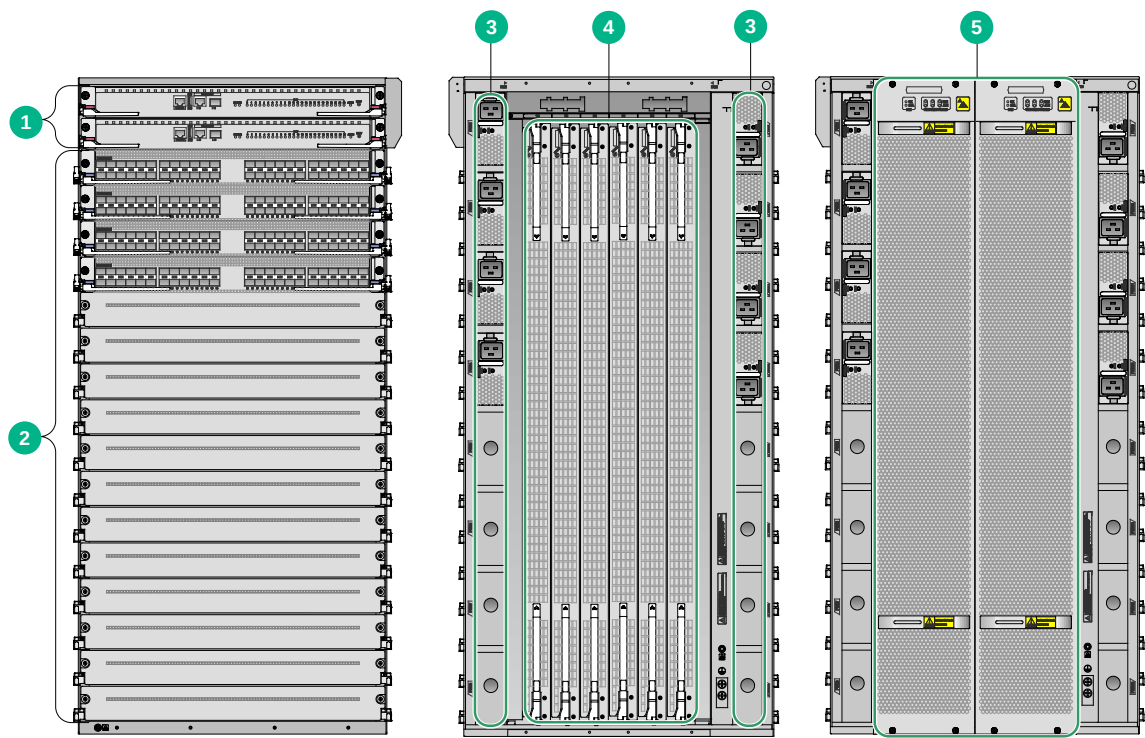
图1-3 S12516G-AF 交换机前、后面板示意图
