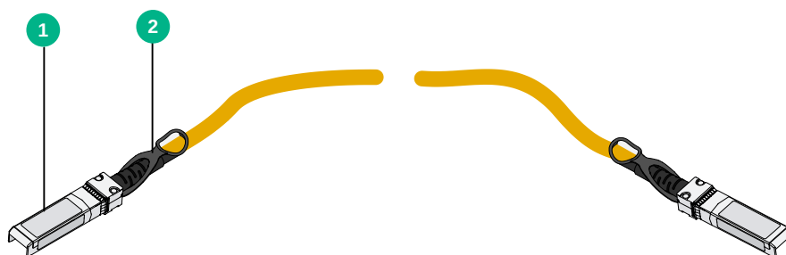
图4-8 SFP28 AOC 光缆示意图
